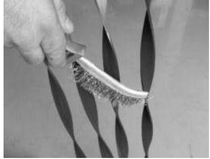
Figura 32 - Limpeza dos canais de passagem de ar e turbuladores
